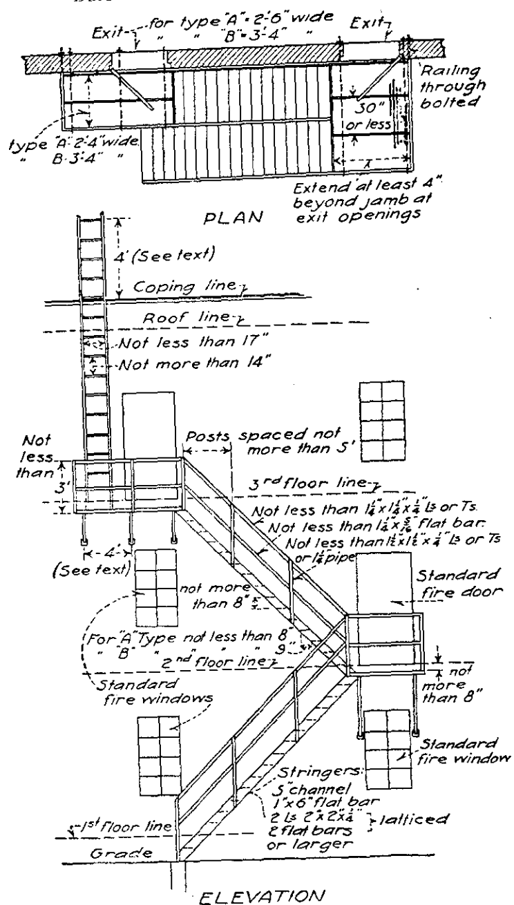
FIRE ESCAPES
